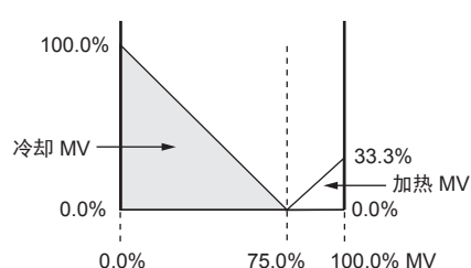
图4 死区=0.0% 加热冷却控制切换点=75.0%的场合
