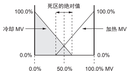
图3 死区<0.0% 加热冷却控制切换点=50.0%的场合
